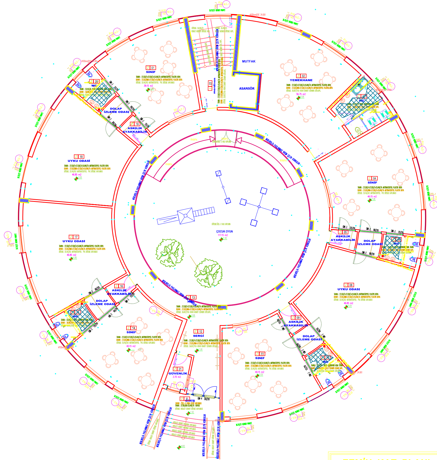
ZEMİN KAT PLANI ÖLÇ.:1/50
